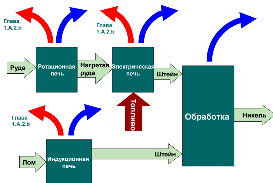
Рисунок 0-1 Упрощенная схема процесса для производства первичного (сверху) и вторичного (снизу) никеля
