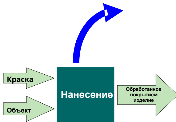
Рисунок 2-1 Технологическая схема для категории источника 2.D.3.d Нанесение покрытия (применяется к подразделам 2.D.3.d.1, 2.D.3.d.2 и 2.D.3.d.3)
