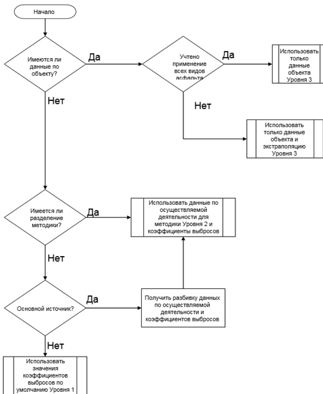
Рисунок 3-1 Дерево решений для категории источника 2.A.6 Асфальтирование дорожного полотна
