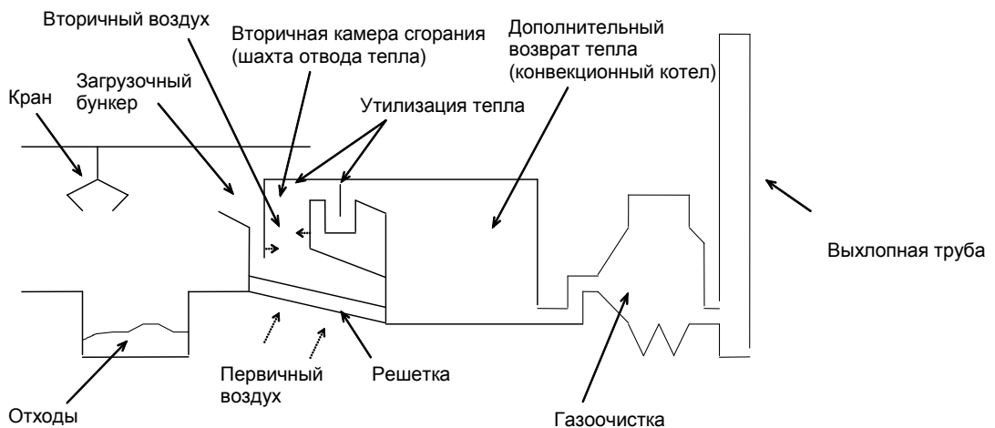
Рисунок 2-2 Компоненты типового инсинератора для массового сжигания коммунально-бытовых отходов с подачей избыточного воздуха
