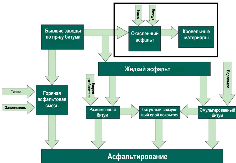
Рисунок 2.1 Обзор производства и использование асфальта. В данной главе рассматриваются все виды деятельности, показанные на рисунке, кроме деятельности, окруженной рамкой в верхней части справа.
