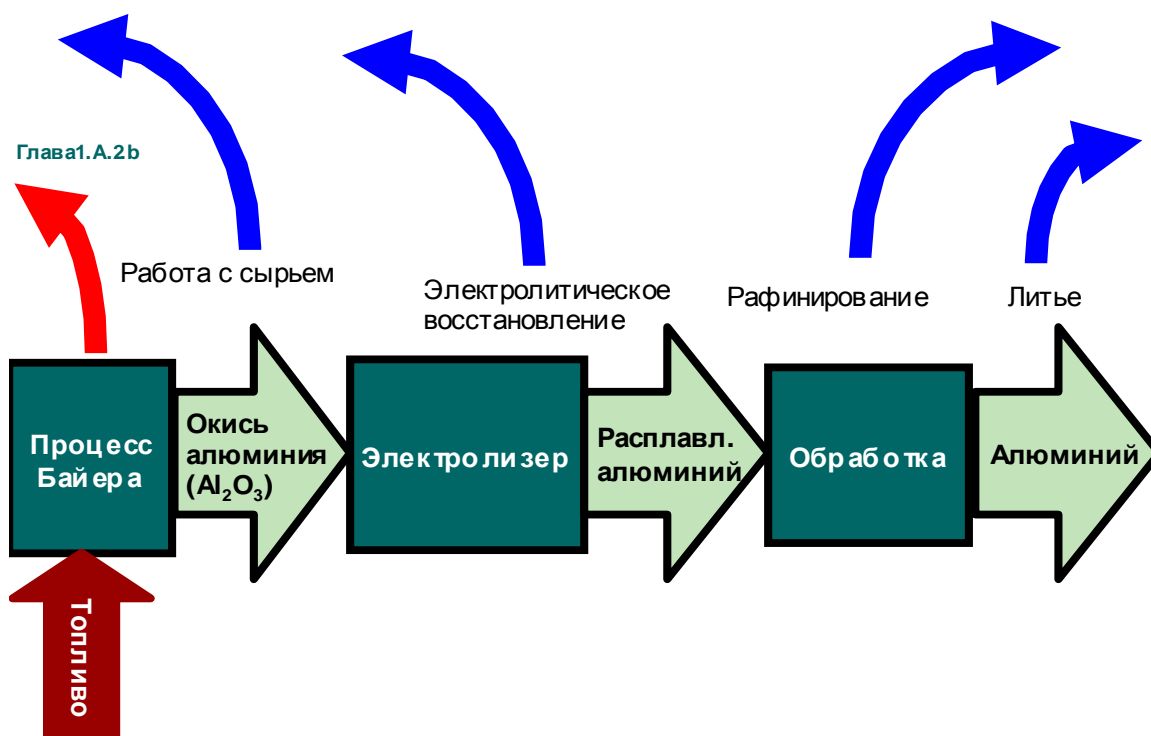
Рисунок 2.1 Схема процесса производства первичного алюминия
