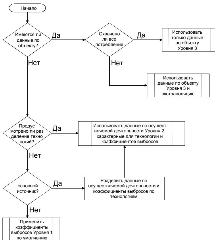
Рисунок 3.1 Дерево решений для категории источников 2.С.3 Производство алюминия.
