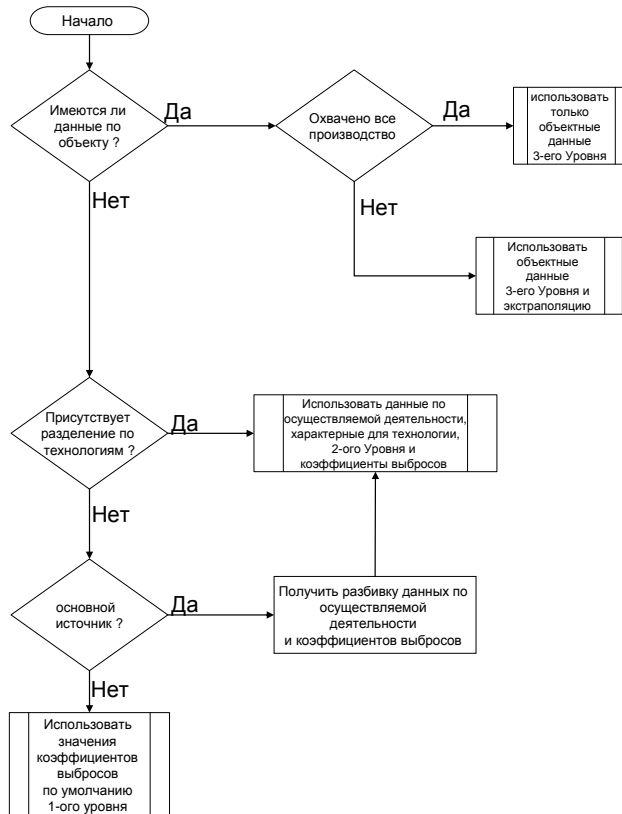
Рисунок 3-1 Схема процесса для категории 6.В Переработка сточных вод
